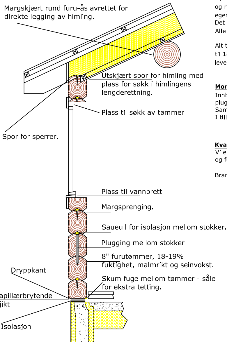
Figur: viser snitt av laftevegg med lafte tekniske detaljer. Her vist med sperretak med krysslufing og 250 mm isolasjon og ringmurs element med støpt isolert såle. opplekket med 48x48 mm og gulv. Mur, såle, gulv, tak konstruksjon og vindu tegnet på figur er ikke med i levering av laftekasse.
