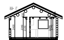
Snitt A-A
