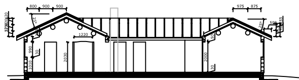
Snitt C-C
